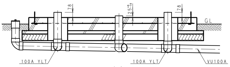
A-A 断面
